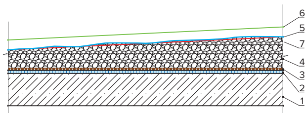
Рис. 5. Неровность уплотненного слоя
