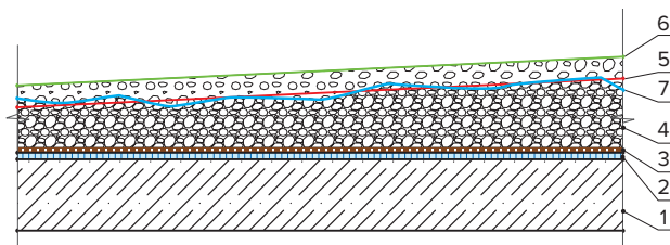
Рис. 10. Определение степени уплотнения слоя ЩП
