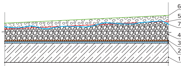
Рис. 9. Определение ровности поверхности
