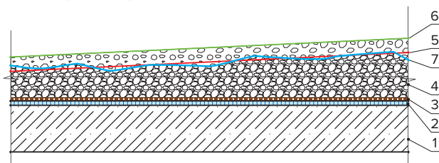
Рис. 4. Неравномерная плотность насыпного слоя
